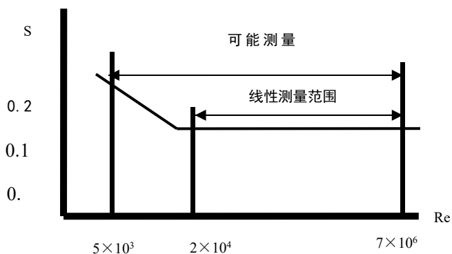
原理图 2
