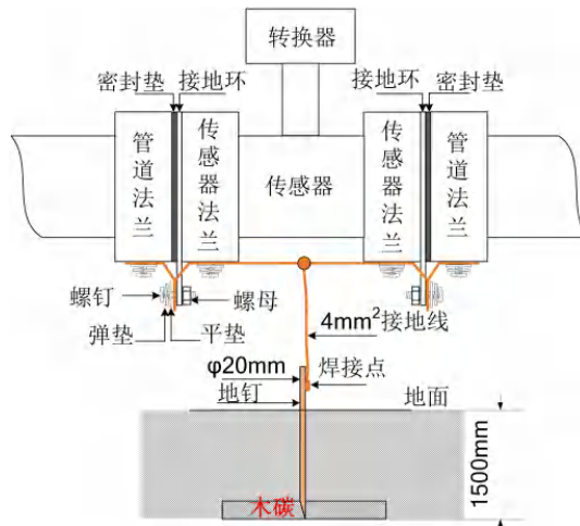
图 1.7 转换器接地示意图
