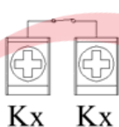
常闭输出
