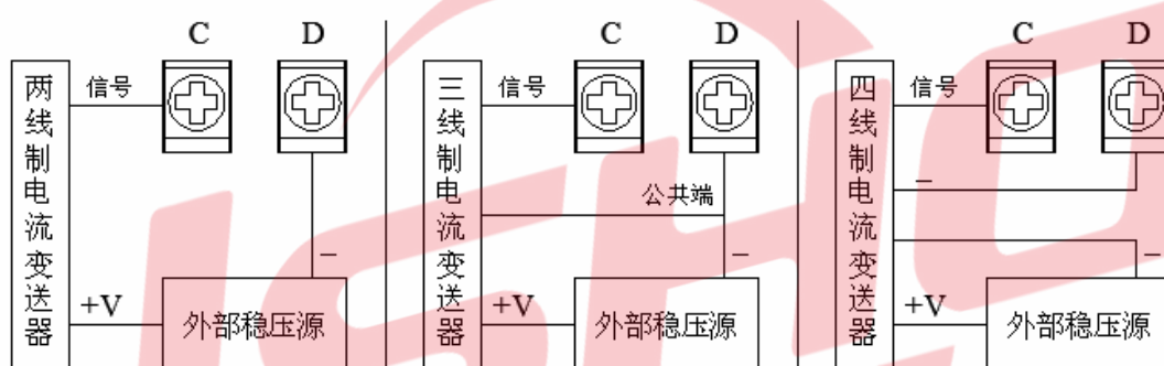
变送器接线方式 (外接稳压源)
