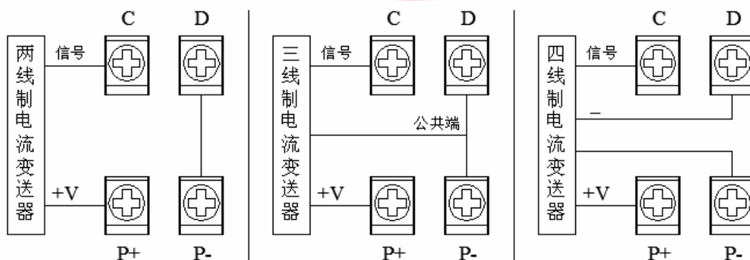
变送器接线方式 (仪表馈电)
