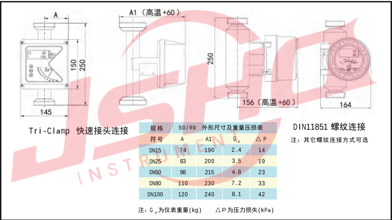
d、50 系列卫生级抛光管外形尺寸及重量压损表
