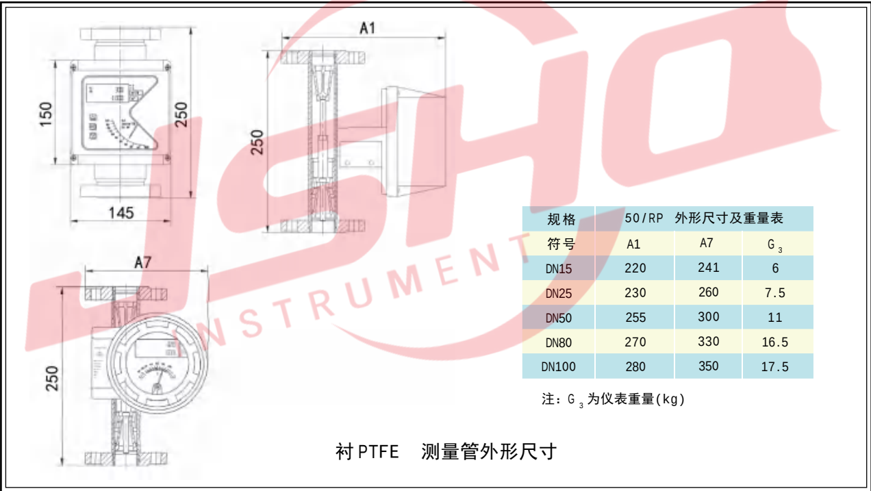
c、50 系列衬 PTFE 型外形尺寸及重量表
