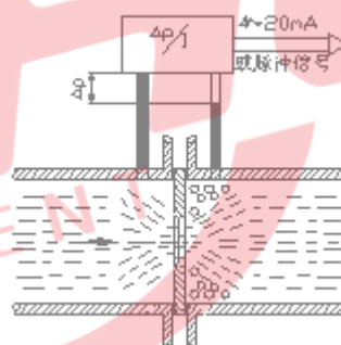
图 2 测量原理示意图
