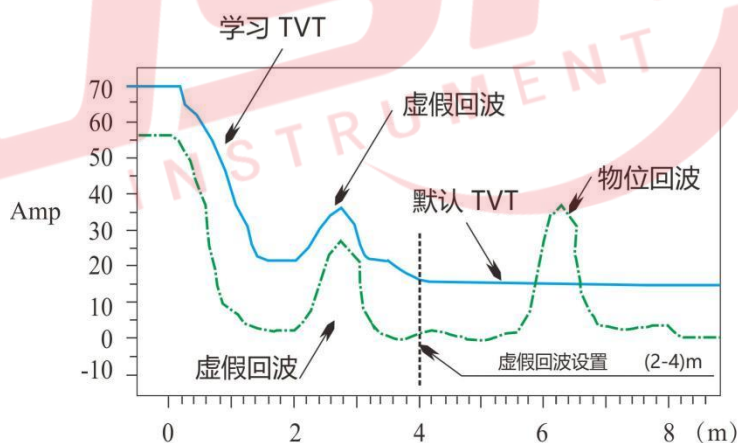
虚拟回波学习后示意图
