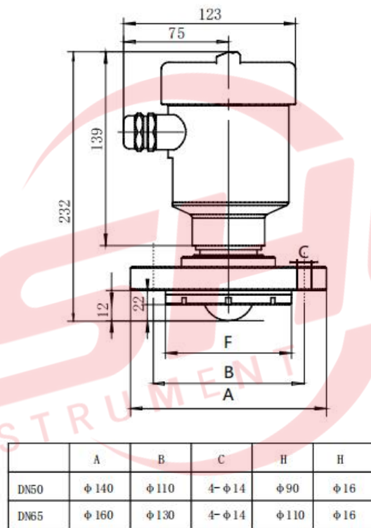
图 3 - 5 防腐法兰常温常压结构尺寸示意图
