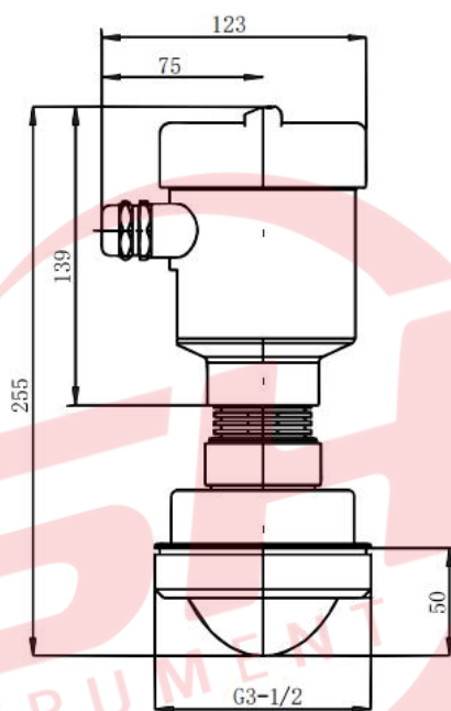
图 3 - 2 管螺纹过程连接高温结构尺寸示意图
