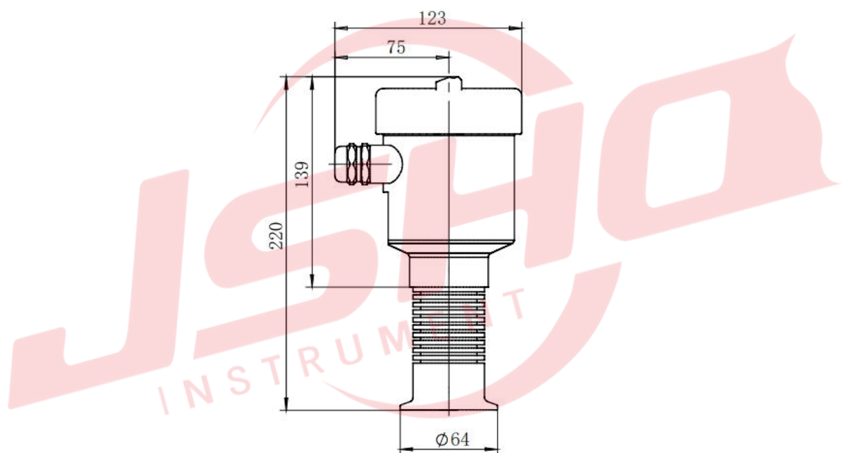
图 3 - 7 卫生卡盘结构尺寸示意图
