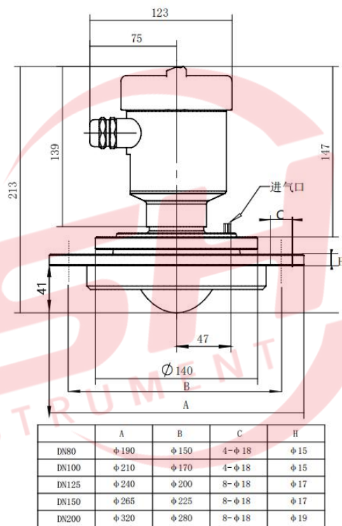
图 3 - 3 万向法兰常温结构尺寸示意图
