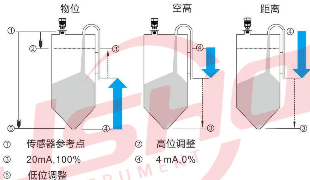
图 6 - 17 电流输出函数示意图
