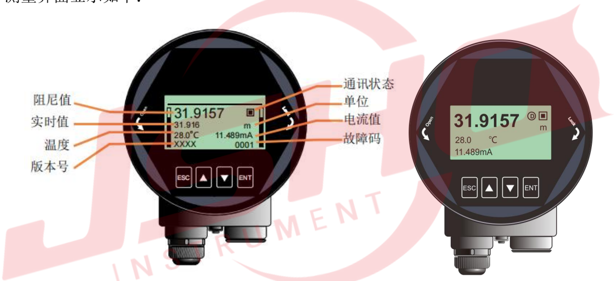
图 6 - 1 测量界面示意图
