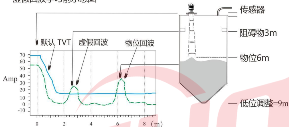
虚拟回波学习前示意图
