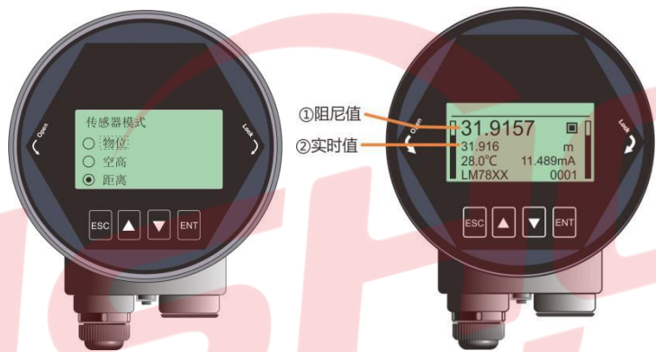
图 6 - 9 传感器模式编辑界面
