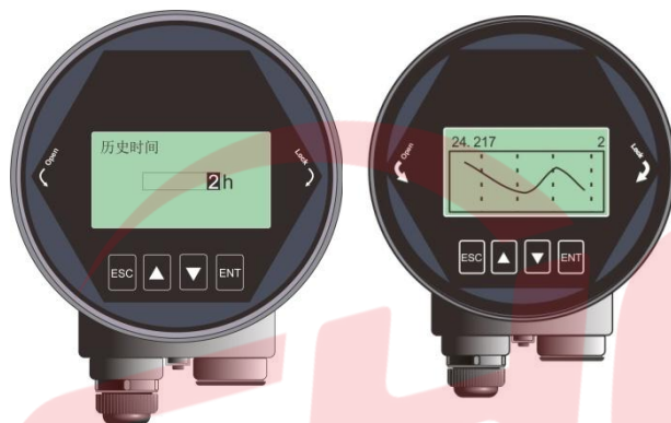
图 6 - 22 历史曲线显示界面
