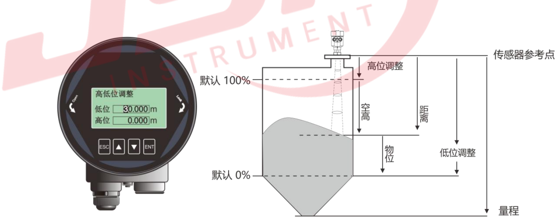
图 6 - 5 低位调整编辑界面与定义
