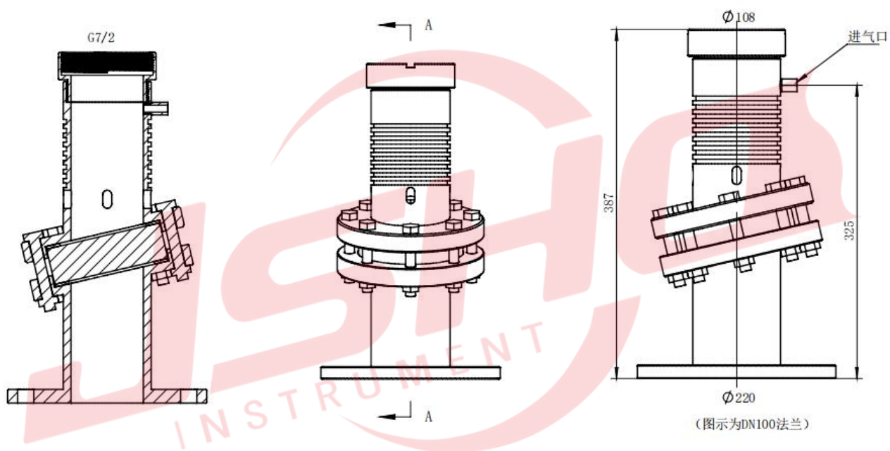
图 3 - 8 高温结构尺寸示意图
