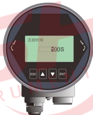
图 6 - 21 丢波时间编辑界面
